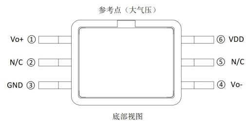
图 3. 引脚定义图
