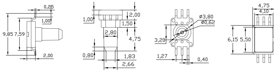
图 1. 外形结构
