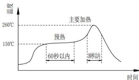
图 5. 回流焊接
