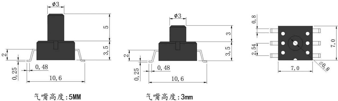
图 1.外形结构
