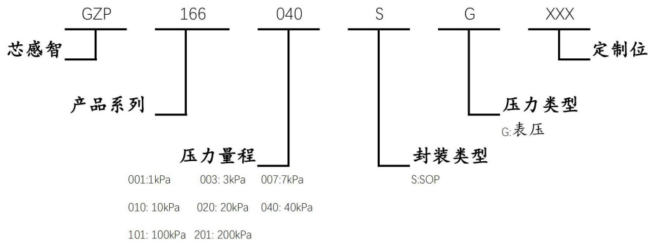
图 2. 选型指南
