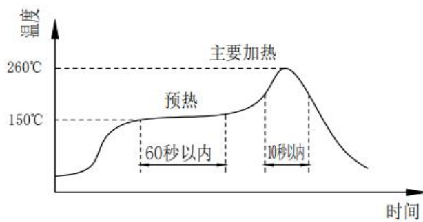
图 3. 回流焊接
