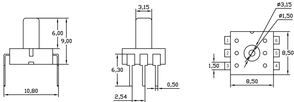
图 2. 外形结构 (DIP 封装形式-R 型)
