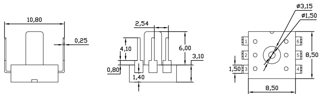
图 3. 外形结构 (DIP 封装形式-F 型)
