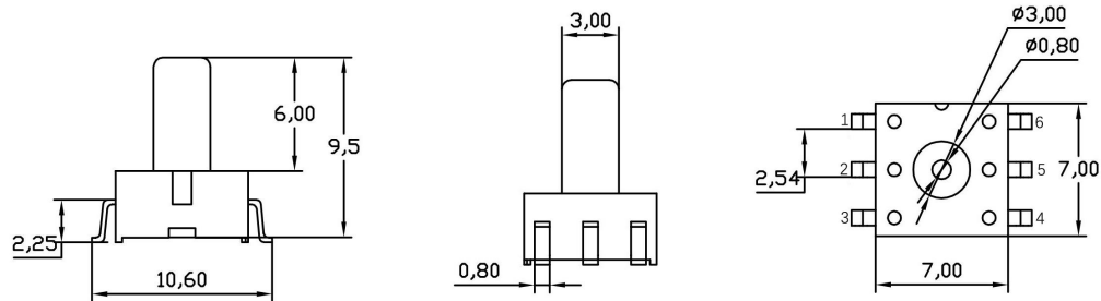
图 1. 外形结构 (SOP 封装形式)
