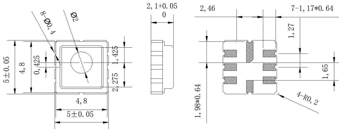
图 1. 外形结构
