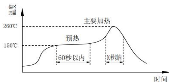
图 3. 回流焊接
