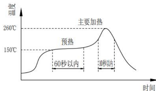
图 5. 回流焊接
