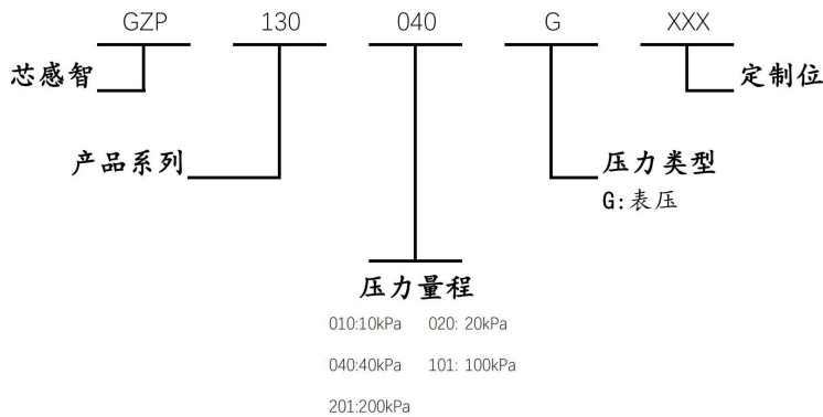
图 4. 选型指南
