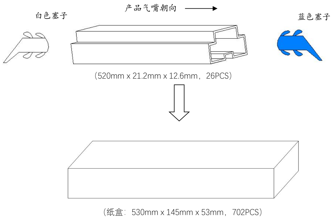
图 8. 包装示意图
