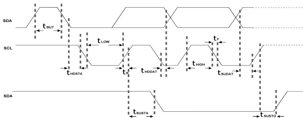
图 3.I 2 C 时序图
