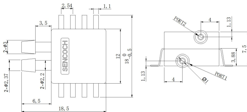
图 1.外形结构
