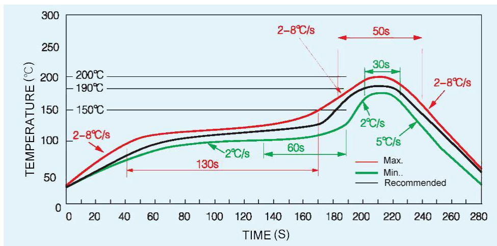
图 6.回流焊接
