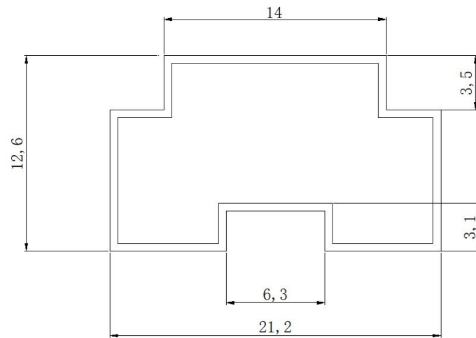
图 7. 料管截面示意图
