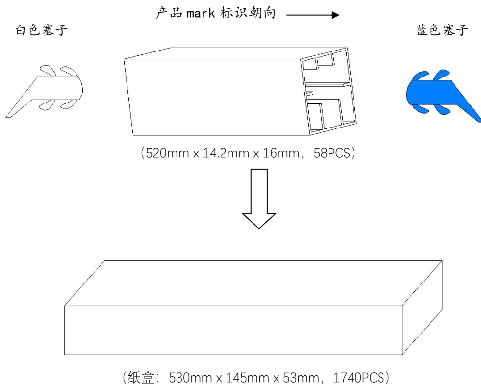
图 13. 包装示意图
