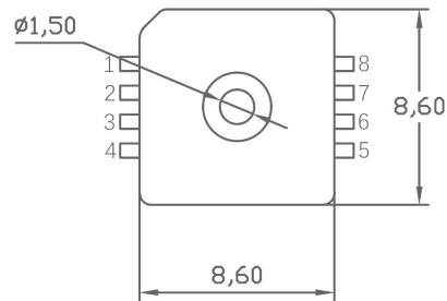
图 5. Top view
