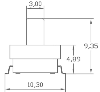
图 3. Side view
