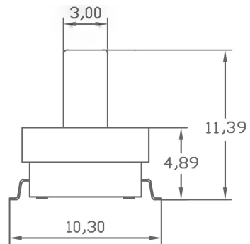
图 6. Side view
