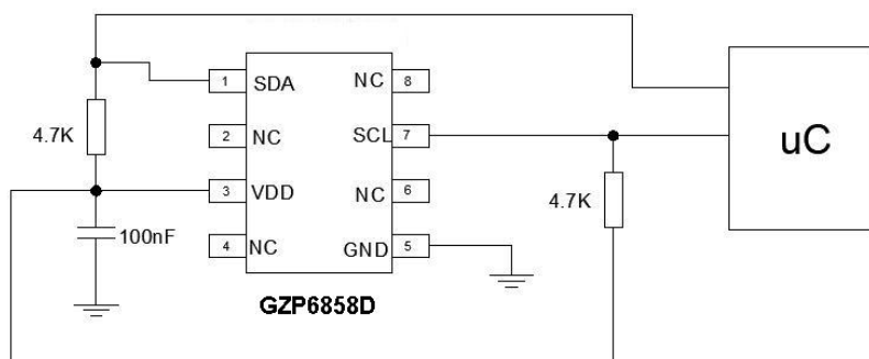
图 7. 典型应用
