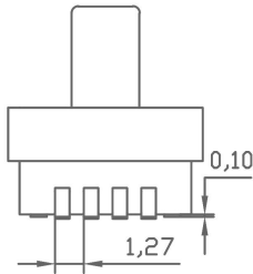
图 1.Side view(引脚面)
