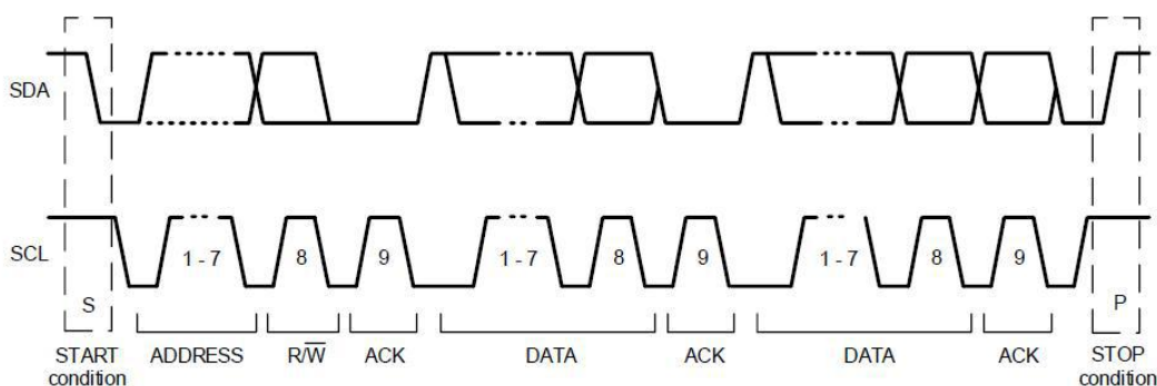
图 9. I 2 C 协议
