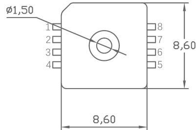
图 2. Top view
