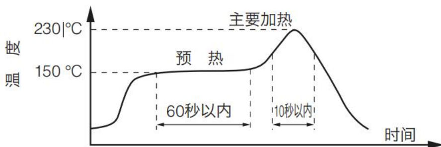
图 11.回流焊接
