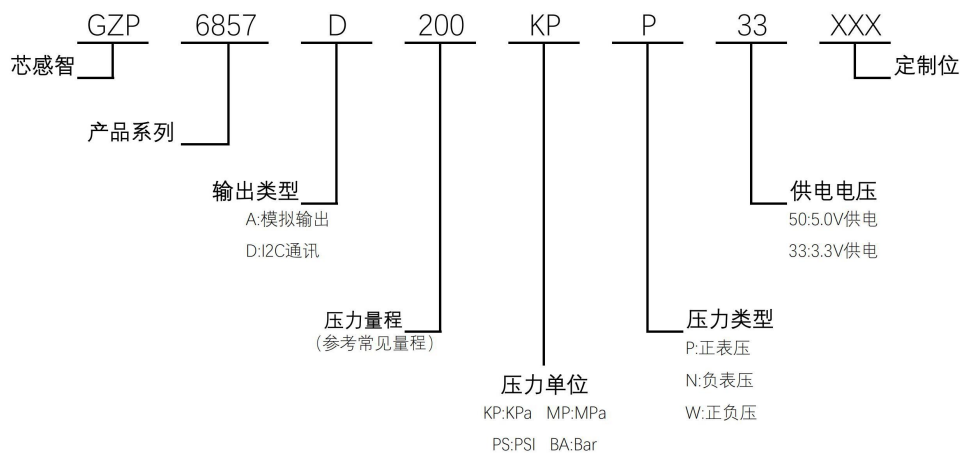
图 5.选型指南
