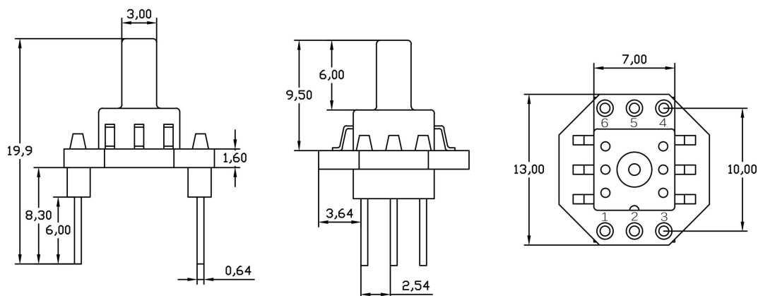
图 1. 外形结构
