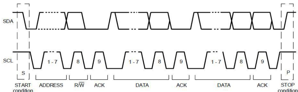
图 4. I²C 协议
