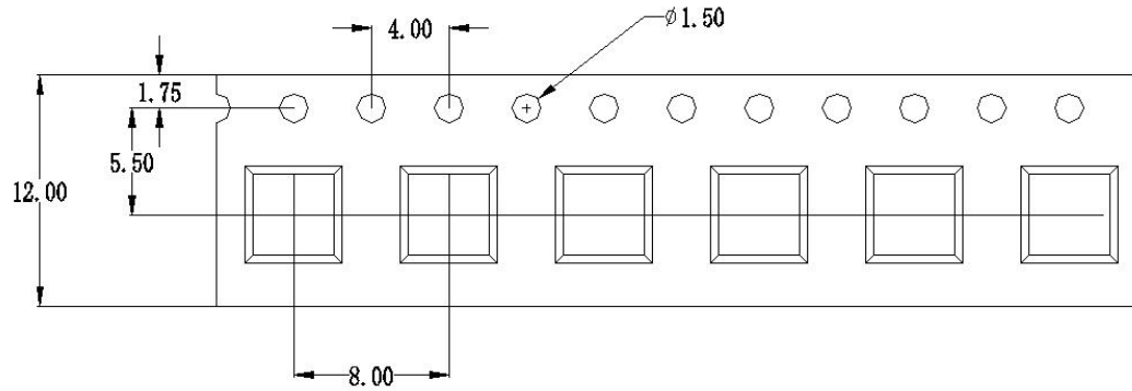
图 5. 载带
