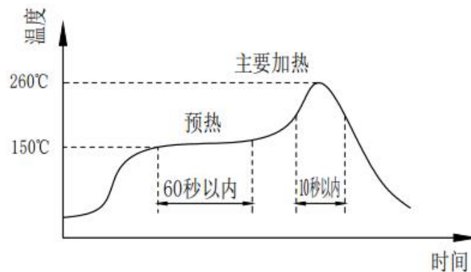
图 4.回流焊接
