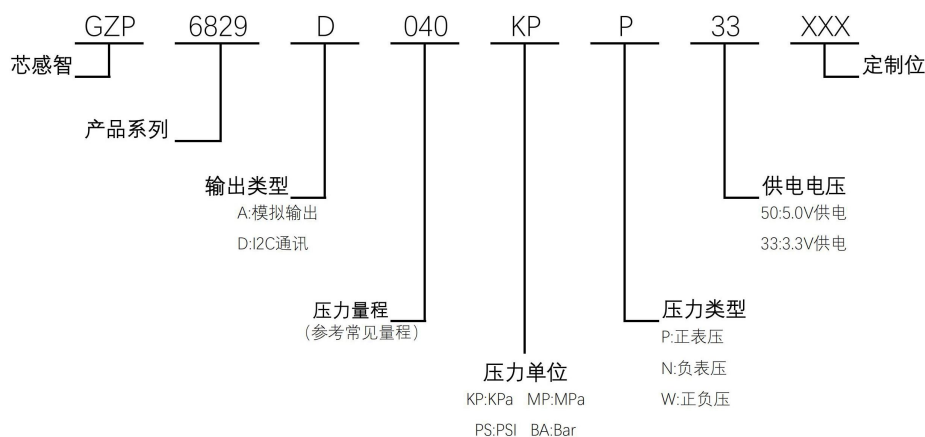
图 3.选型指南
