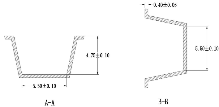
图 6. 载带口袋细节图
