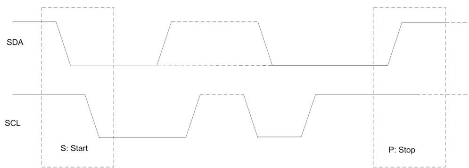
图 2.IIC 时序图
