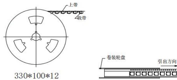
图 7. 载带转盘
