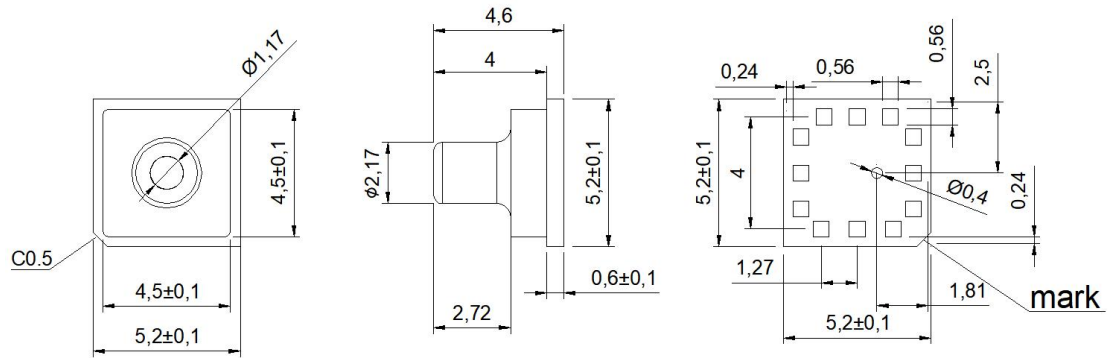
图 1.外形结构
