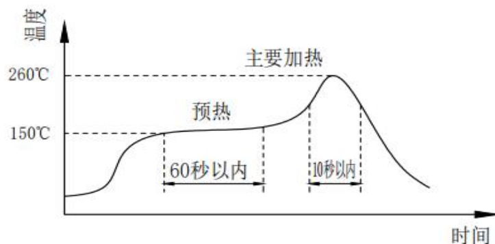
图 4.回流焊接
