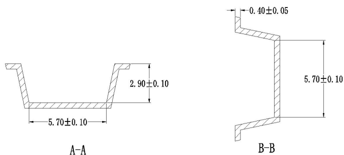
图 6. 载带口袋细节图
