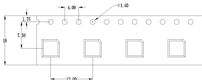
图 5. 载带
